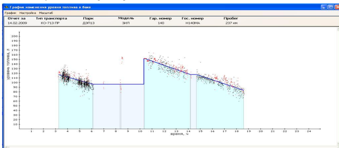
Рисунок В.1 - График изменения уровня топлива по указанной машине за указанный период времени, построенный по данным, передаваемым от датчика уровня топлива машины.
